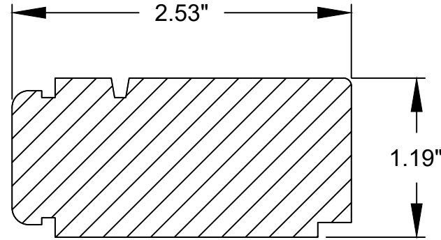
JAMB FRAME (PINE)
